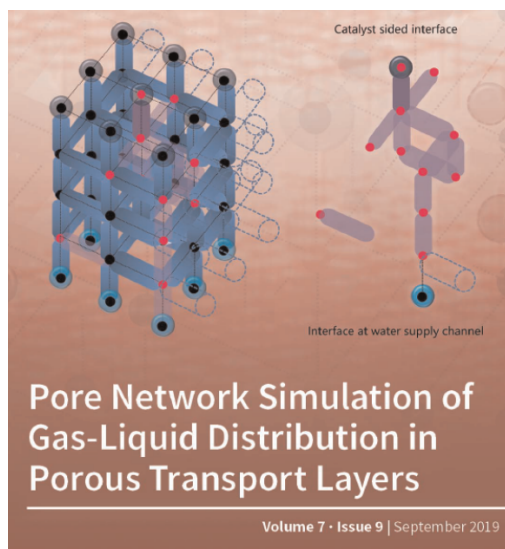
Abbildung 8. Deckblatt der Zeitschrift Processes aus [20]. Links: Schematische Illustration eines Porennetzwerkes für die Drainage der Transportschicht an der Anode einer Wasserelektrolyse (Poren in blau, Porenhälse in schwarz). Rechts: Pfad bei Durchbruch des Sauerstoffs von der Katalysatorseite zum Wasserversorgungskanal.
