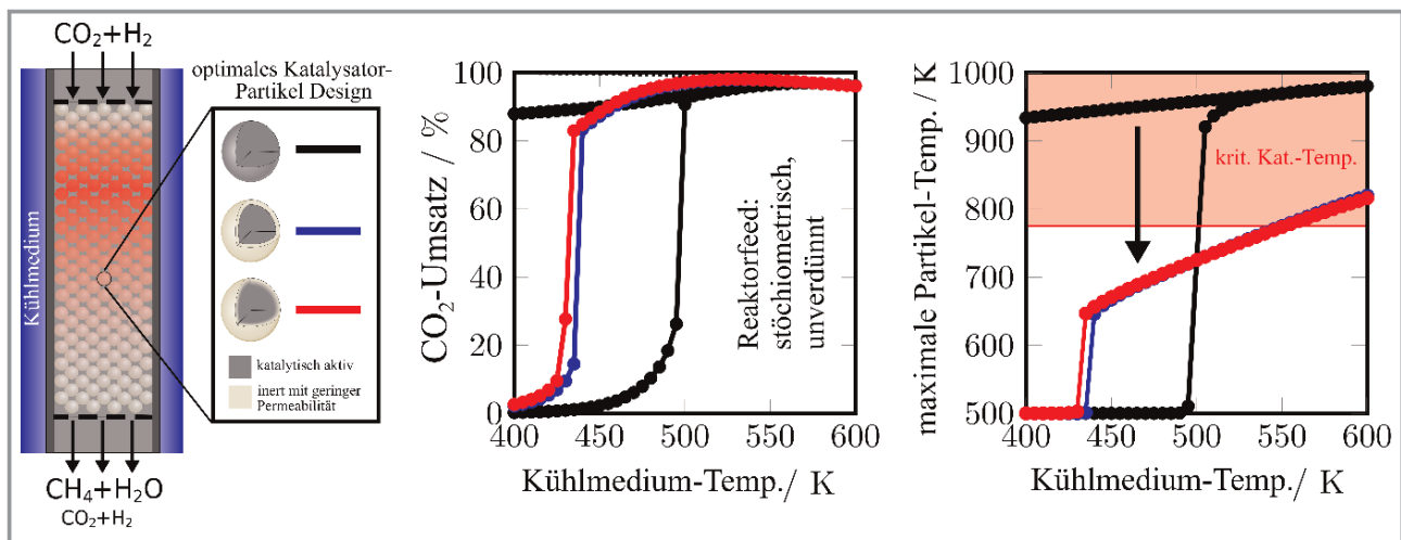
Abbildung 6. Die thermische Sensitivität der stark exothermen \text{CO}_2 -Methanisierung in Festbettreaktoren lässt sich durch den Einsatz eines maßgeschneiderten Katalysators, der einen aktiven Kern und eine dünne poröse Inerthülle besitzt, deutlich reduzieren [15].
