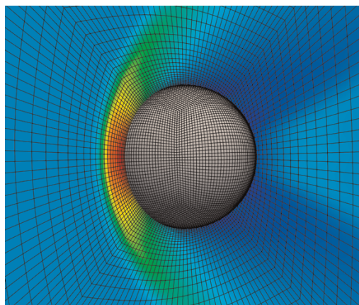
Abbildung 10. Simulation einer stehenden Stoßwelle vor einem Partikel bei Machzahl 2.
