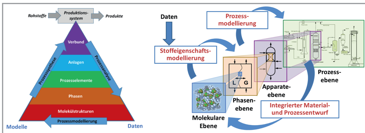
Abbildung 5. Das Forschungskonzept des Lehrstuhls Systemverfahrenstechnik beruht auf der Analyse und Synthese von Produktionssystemen auf fünf hierarchischen Ebenen (links). Datengetriebene und mechanistische Modelle werden miteinander verknüpft, um den integrierten Material-Prozess-Entwurf zu unterstützen (rechts).
