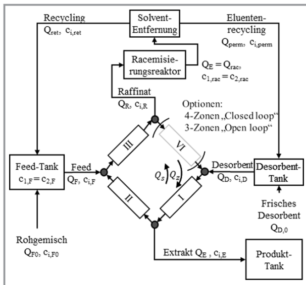
Abbildung 4. Kopplung von kontinuierlicher SMB-Chromatographie mit enzymatischer Racemisierung zur verlustfreien Gewinnung von reinen Enantiomeren aus racemischen Mischungen [9].
