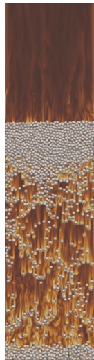
Abbildung 9. Momentaufnahme der Simulation eines vollaufgelösten Wirbelschichtreaktors.
