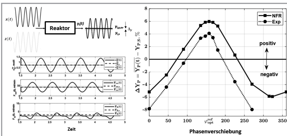
Abbildung 3. Demonstration des Potenzials einer erzwungen dynamischen Betriebsweise von Reaktoren unter Nutzung der periodischen Anregung zweier phasenverschobener Eingangsgrößen (hier des Zulaufstroms und der Eingangszusammensetzung) sowie der Vorhersagekraft der NFR-Methode [7].
