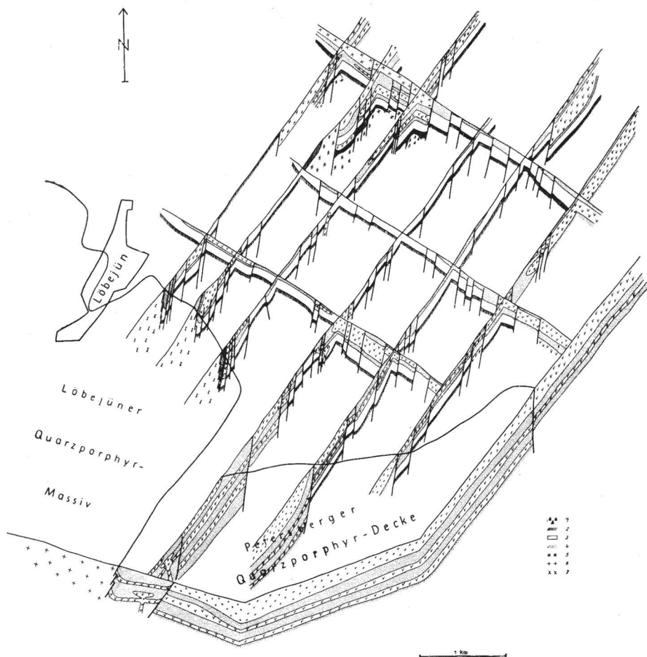
Abb. 6. Schnitte durch die Steinkohlenlagerstätte Plötz 1 Kristalliner Sockel, 2 Mansfelder Schichten, 3 Wettiner Schichten, 4 Hallesche Schichten, 5 Wieskauer Porphyry, 6 Lobejüner Porphyry, 7 Petersberger Porphyry.
