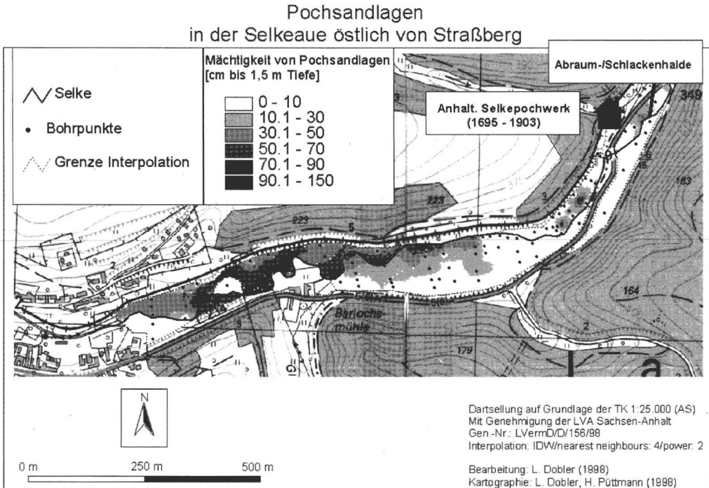
Abb. 7: Verbreitung und Mächtigkeit von Pochsandlagen im Flußabschnitt B2 östlich von Straßberg
