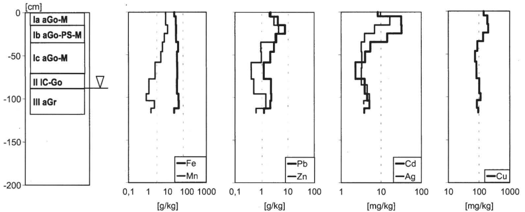
Abb. 6: Profilaufbau und Tiefgradienten der Schwermetalle im Flußabschnitt E
