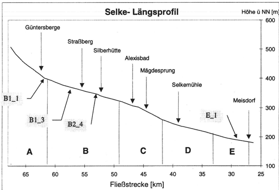
Abb. 2: Längsprofil (Wasserspiegelhöhe) mit Flußabschnitten der Selke im Harz und Lage der Profile
