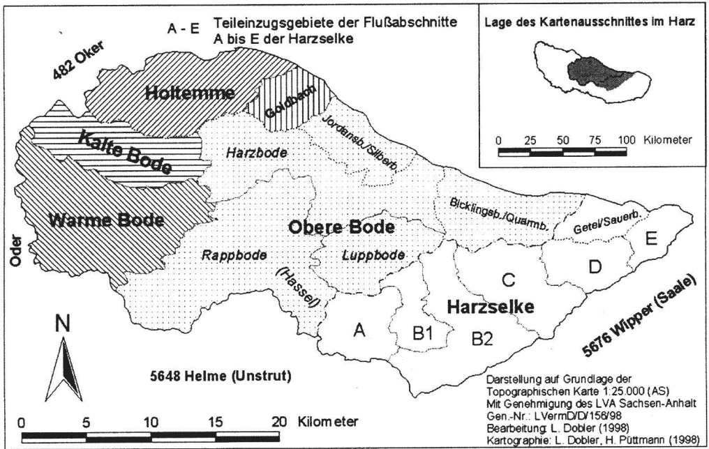
Abb. 1: Oberirdische Wassereinzugsgebiete von Bode und Selke im Harz
