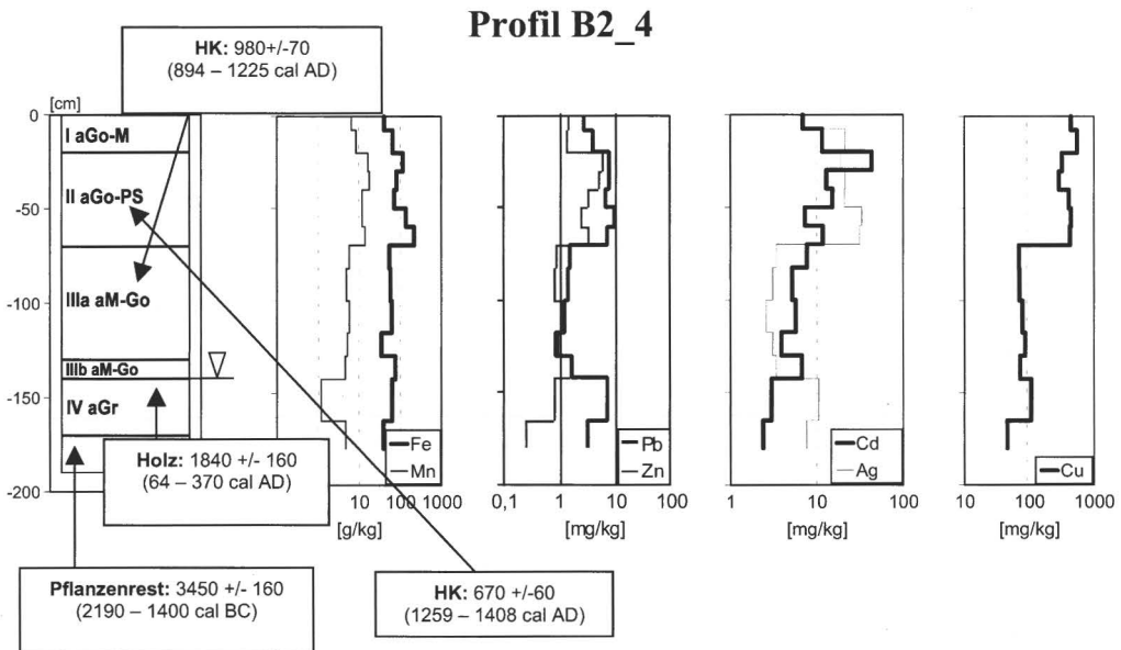
Abb. 4: Profilaufbau und Tiefengradienten der Schwermetalle im Flußabschnitt B2
