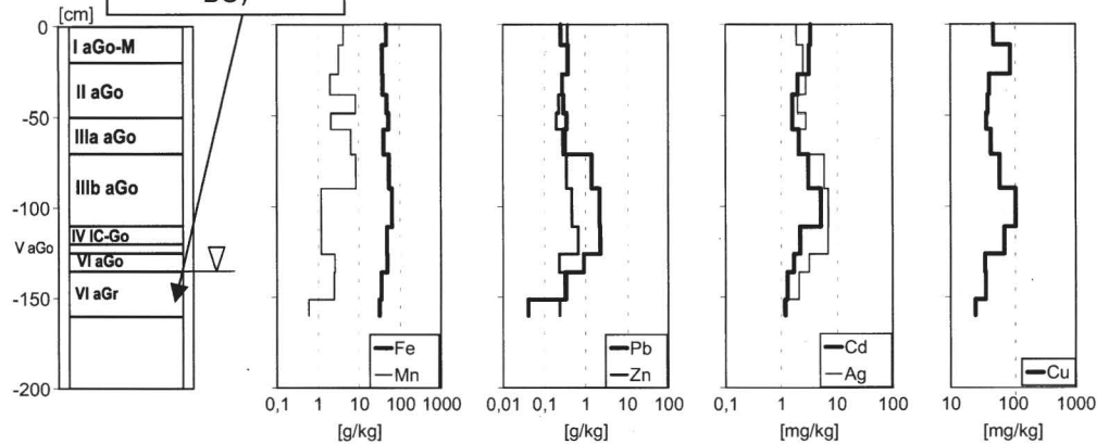
Abb. 3: Profilaufbau und Tiefengradienten der Schwermetalle in ausgewählten Profilen des Flußabschnittes B1
