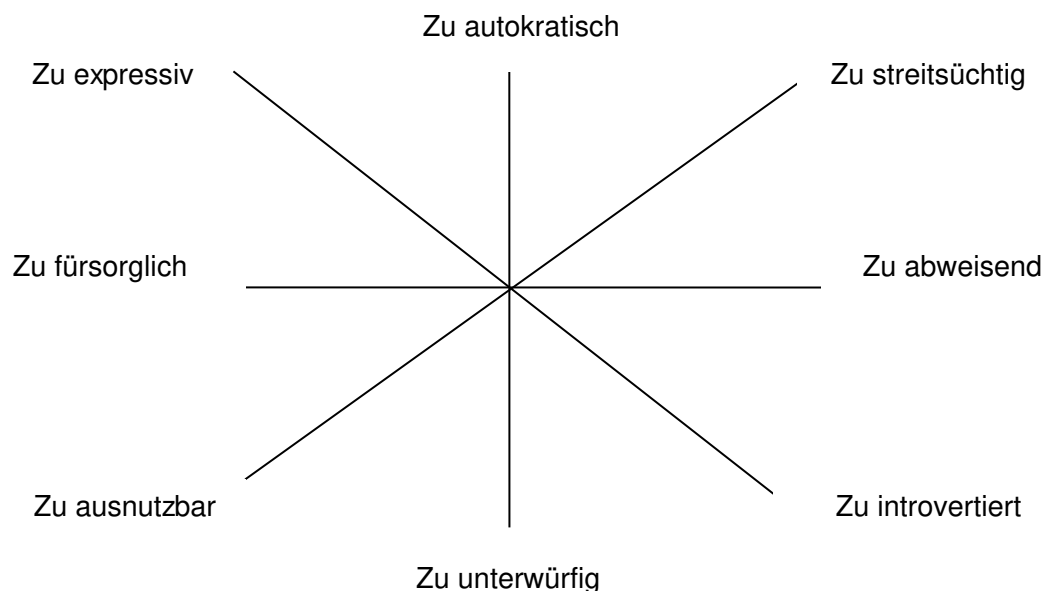
Abbildung 1.1: Zirkumplex-Modell
