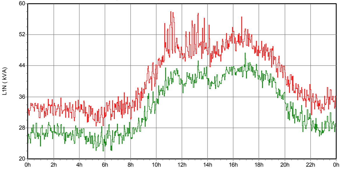
Leistung. Von 17.01.2013 00:00:00 Bis 17.01.2013 23:58:23
