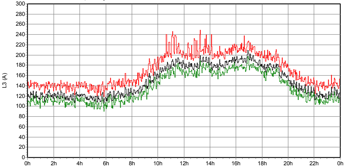
Spannung und Strom. Von 17.01.2013 00:00:00 Bis 17.01.2013 23:58:23
