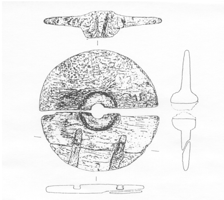
Abb. 8: Scheibenrad von Kideris, Dänemark, mit rundem Achsloch (nach Häusler 1994)
