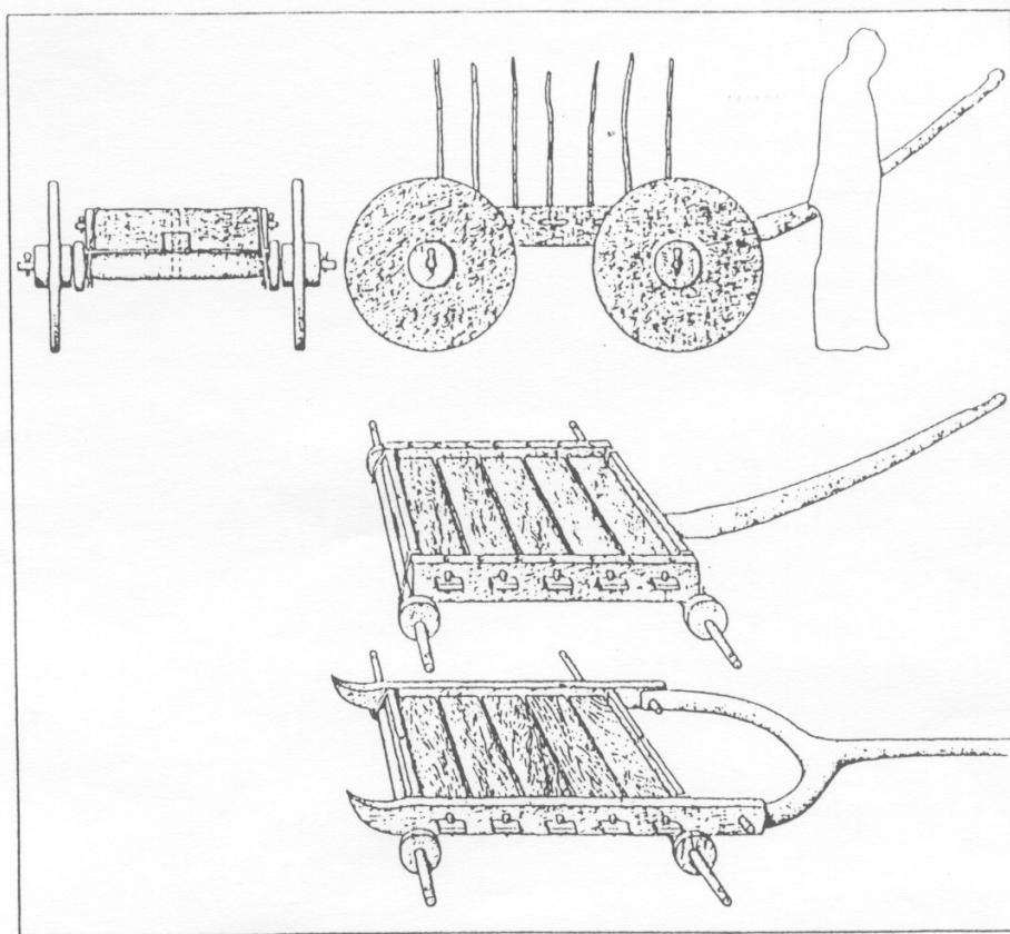
Abb. 13: Rekonstruktion eines neolithischen Wagens (nach Hayen 1989)
